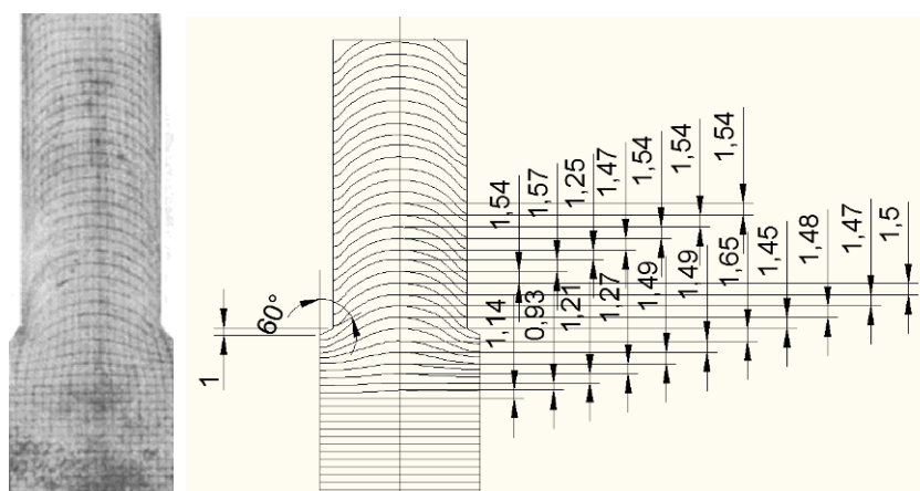
Fig.3 Die grid network 60° x 1mm
