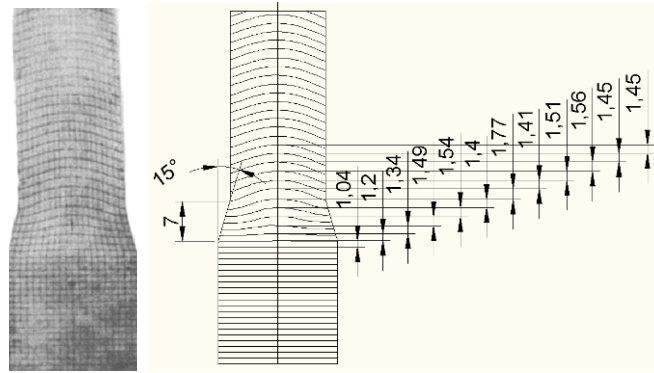
Fig.4 Die grid network 15°x7mm.
