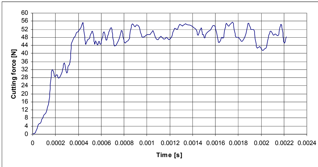
Fig. 3 The cutting force F_z - a_p = 0,5 mm, f = 0,1 mm/rev, v = 58,875 m/min
